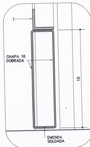
DET. 4 ESC. 1:2.5
