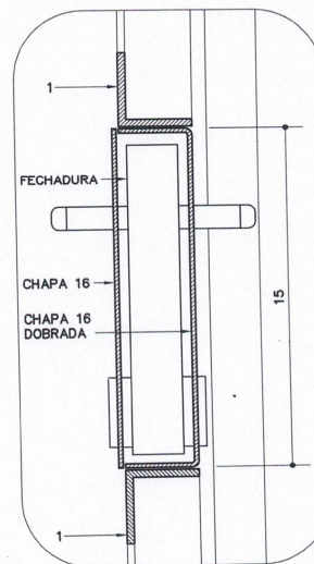
DET. 3 ESC. 1:2.5
