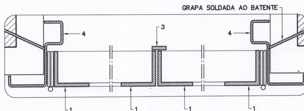
DET. 1 ESC. 1:2.5
