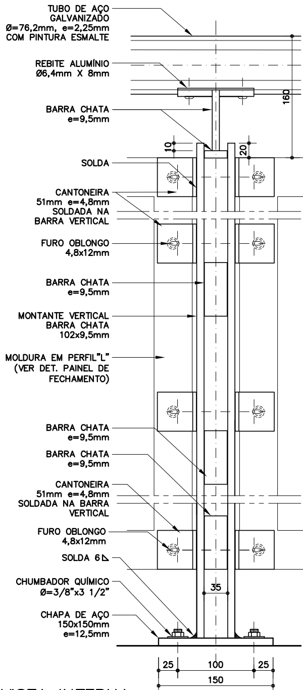
VISTA INTERNA
