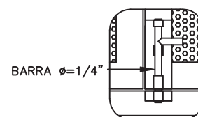
DET. 7 ESC. 1:5 FECHO INFERIOR
