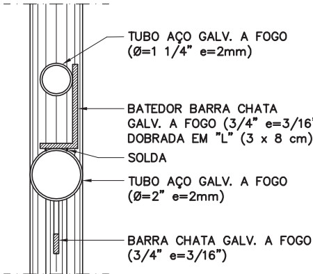
DETALHE DO BATEDOR ESC. 1:5
