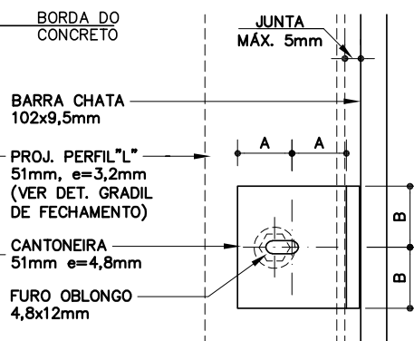
DETALHE CANTONEIRA
