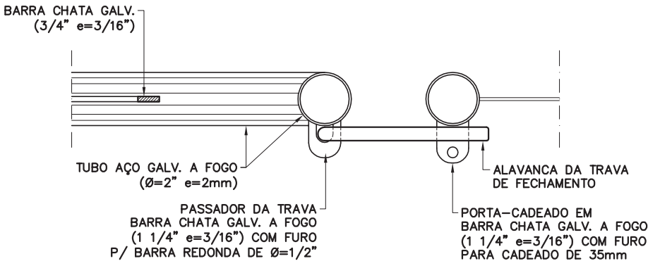
DETALHE 1 ESC. 1:5
