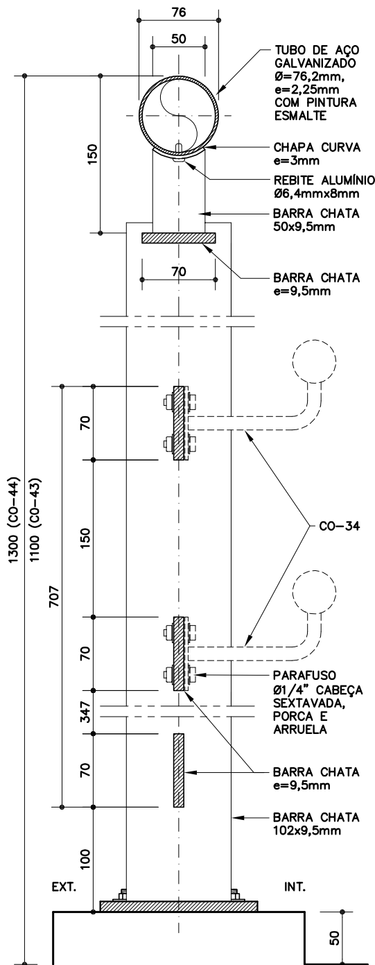
CORTE TRANSVERSAL
