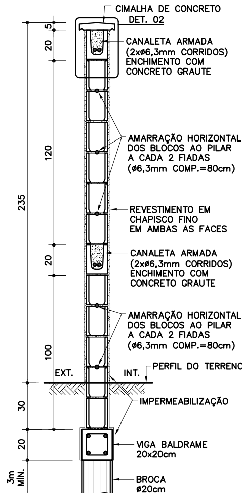
CORTE BB
