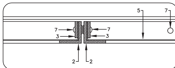
DET. 2 ESC. 1:2,5
