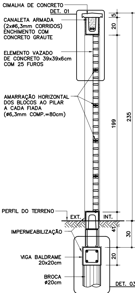
CORTE AA
