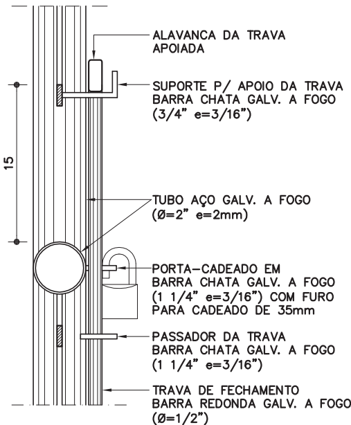
DETALHE 2 ESC. 1:5
