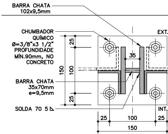
PLANTA BASE DE FIXAÇÃO
