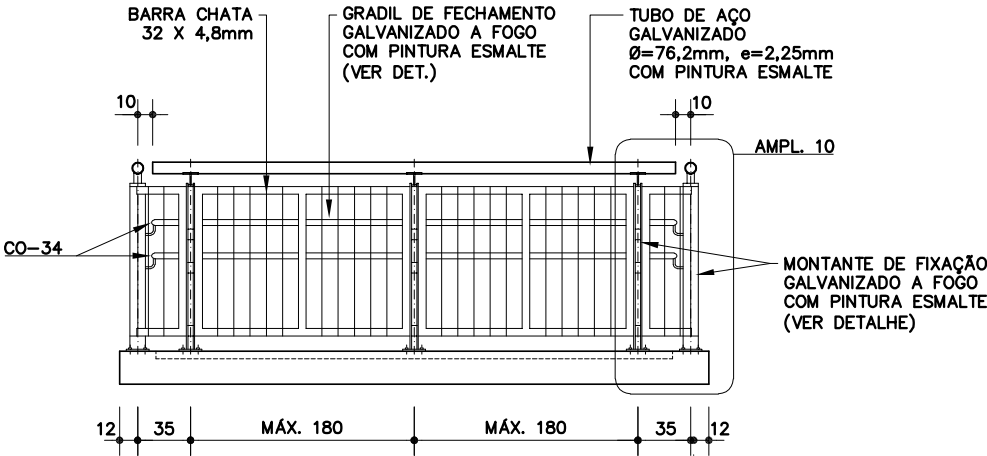
VISTA 1 ESC. 1: 50
