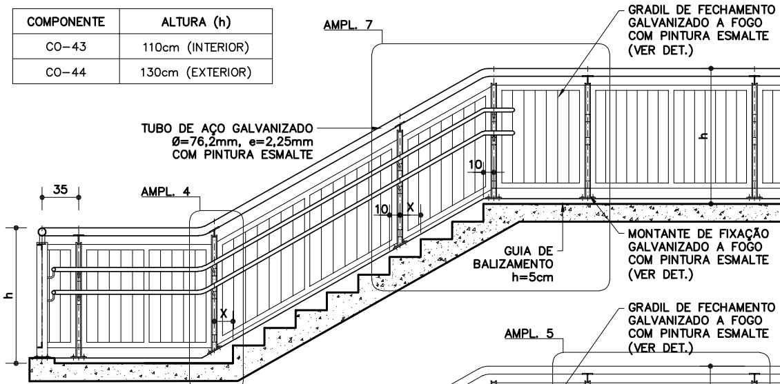
CORTE A ESC. 1:50
