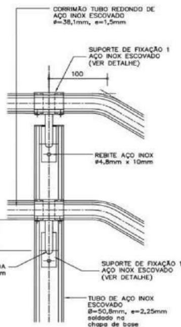
DET. 4 ESC. 1:5 MEDIDAS EM MILÍMETROS
