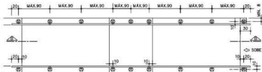
PLANTA GENÉRICA DE RAMPA ESC. 1:50
