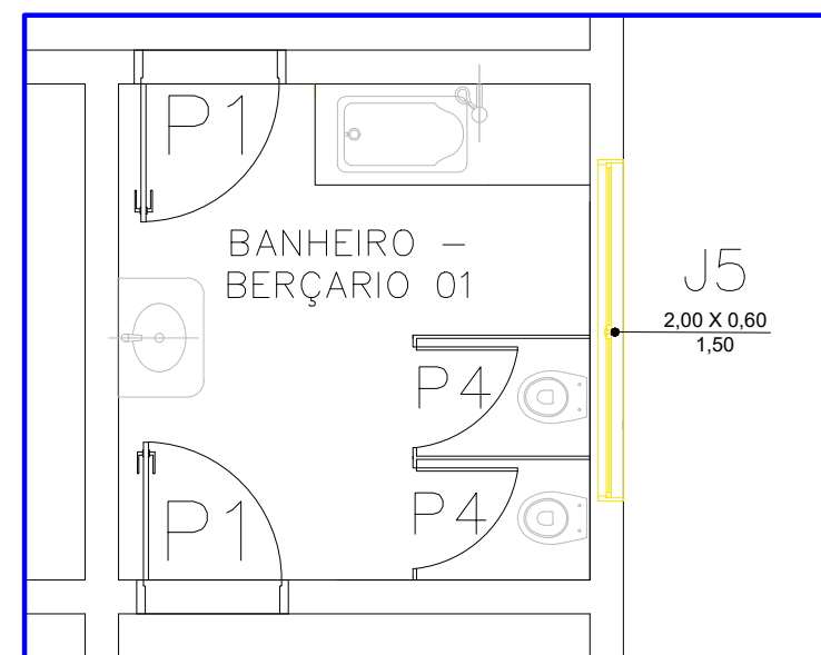
DETALHAMENTO 01 – BANHEIRO BERÇÁRIO 01 ESC: 1/50
