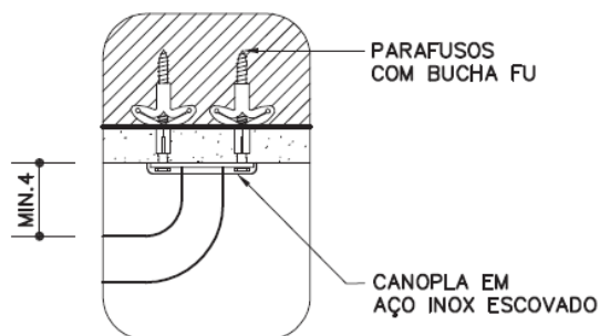
CORTE A-A ESC. 1:20
