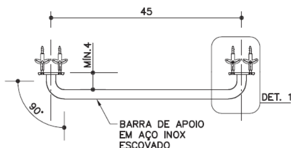
DET. BARRA DE APOIO ESC. 1:10
