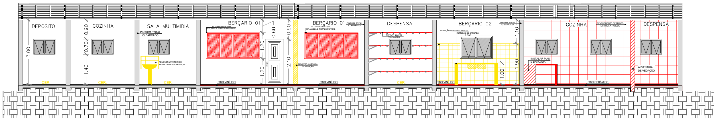
CORTE A–A
