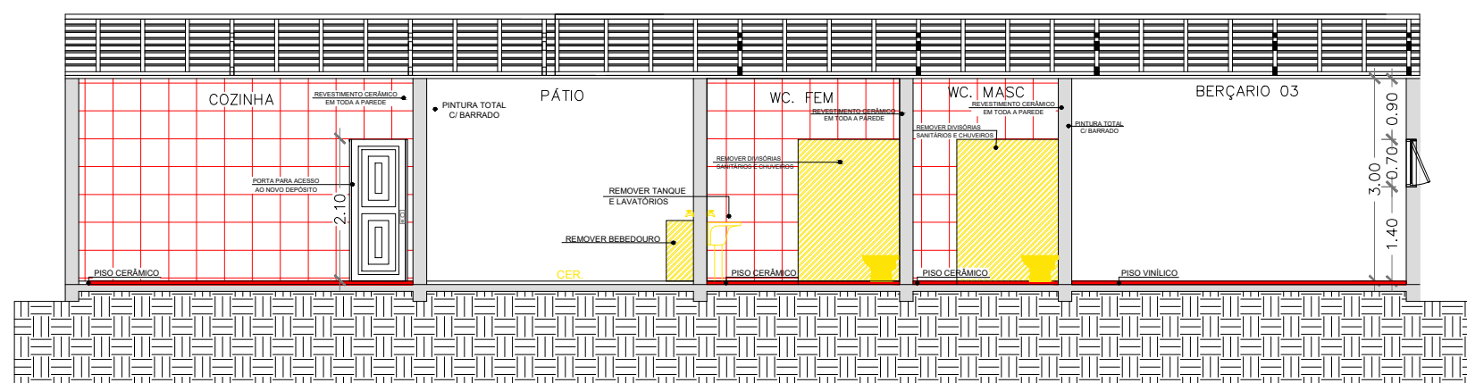
CORTE B–B ESC: 1/100
