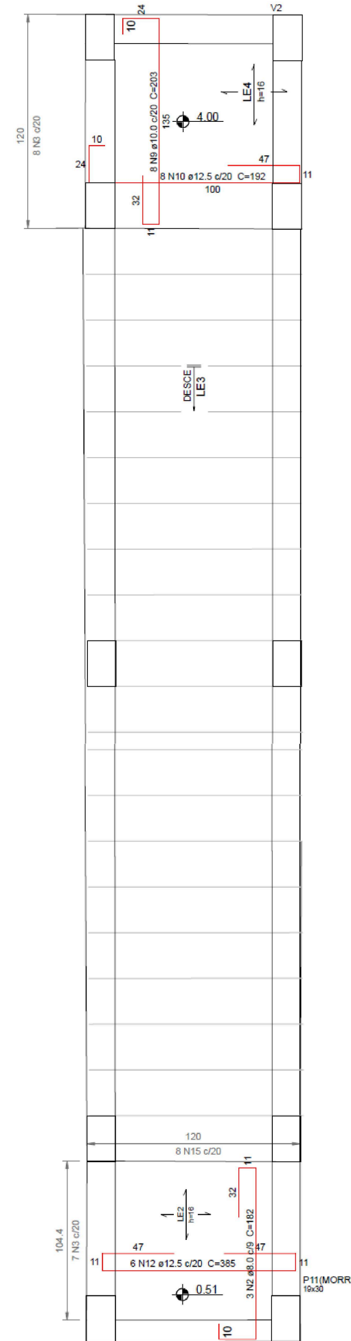
ARMAÇÃO POSITIVA DA ESCADA E1 Escala 1:25
