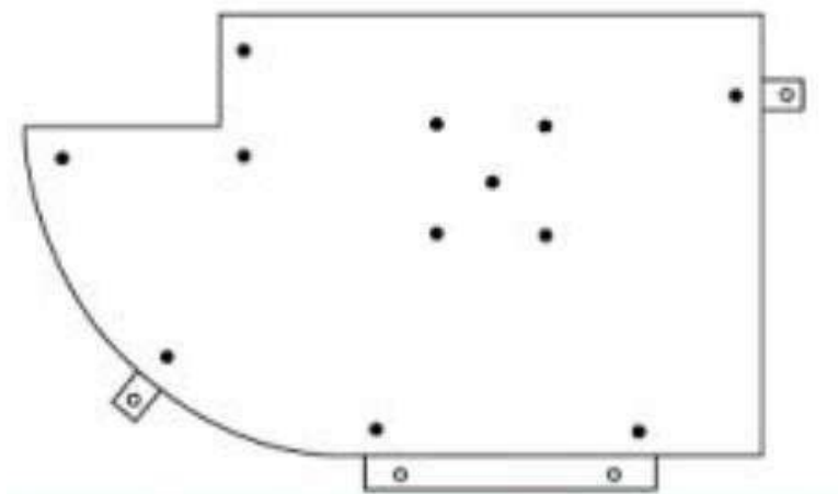
Figura 14 - Área dos disparos (ASTM E3113-18)
