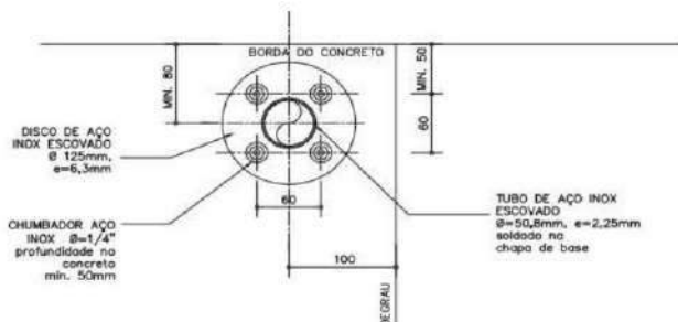
DET. 2 - BASE DE FIXAÇÃO MONTANTE VERTICAL
