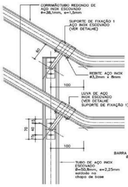
DET. 3 ESC. 1:5 MEDIDAS EM MILÍMETROS
