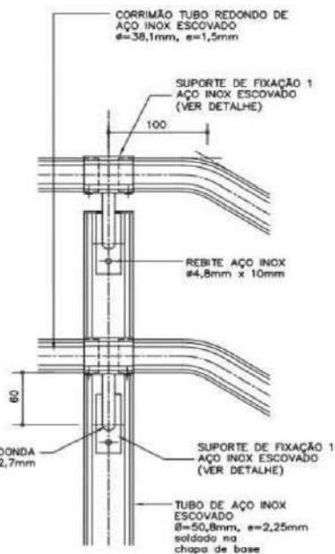
DET. 4 ESC. 1:5 MEDIDAS EM MILÍMETROS
