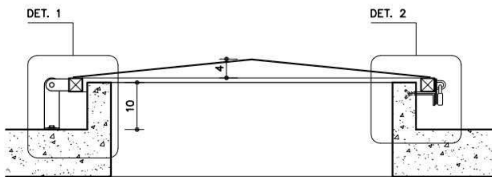
CORTE AA
