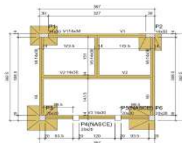
Forma do pavimento PISO
