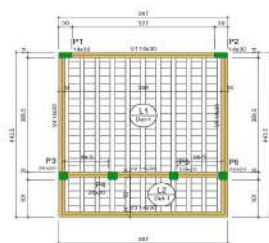
Forma do pavimento COBERTURA
