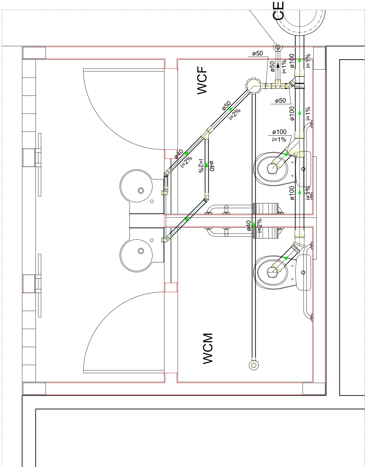
DETALHE SAN-1 1:25
