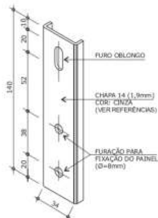
SUPORTE METÁLICO
